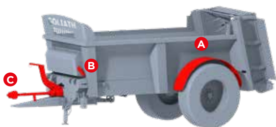
(A) Garde-boue en acier (B) Porte-documents avec livre de pièces personnalisé (C) Porte-flexible et cardan grand angle avec sécurité à cames.
