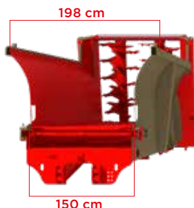
Caisse arrondie pour faciliter l'évacuation de la marchandise, réalisée par croquage de la tôle pour une rigidité accrue des côtés.
